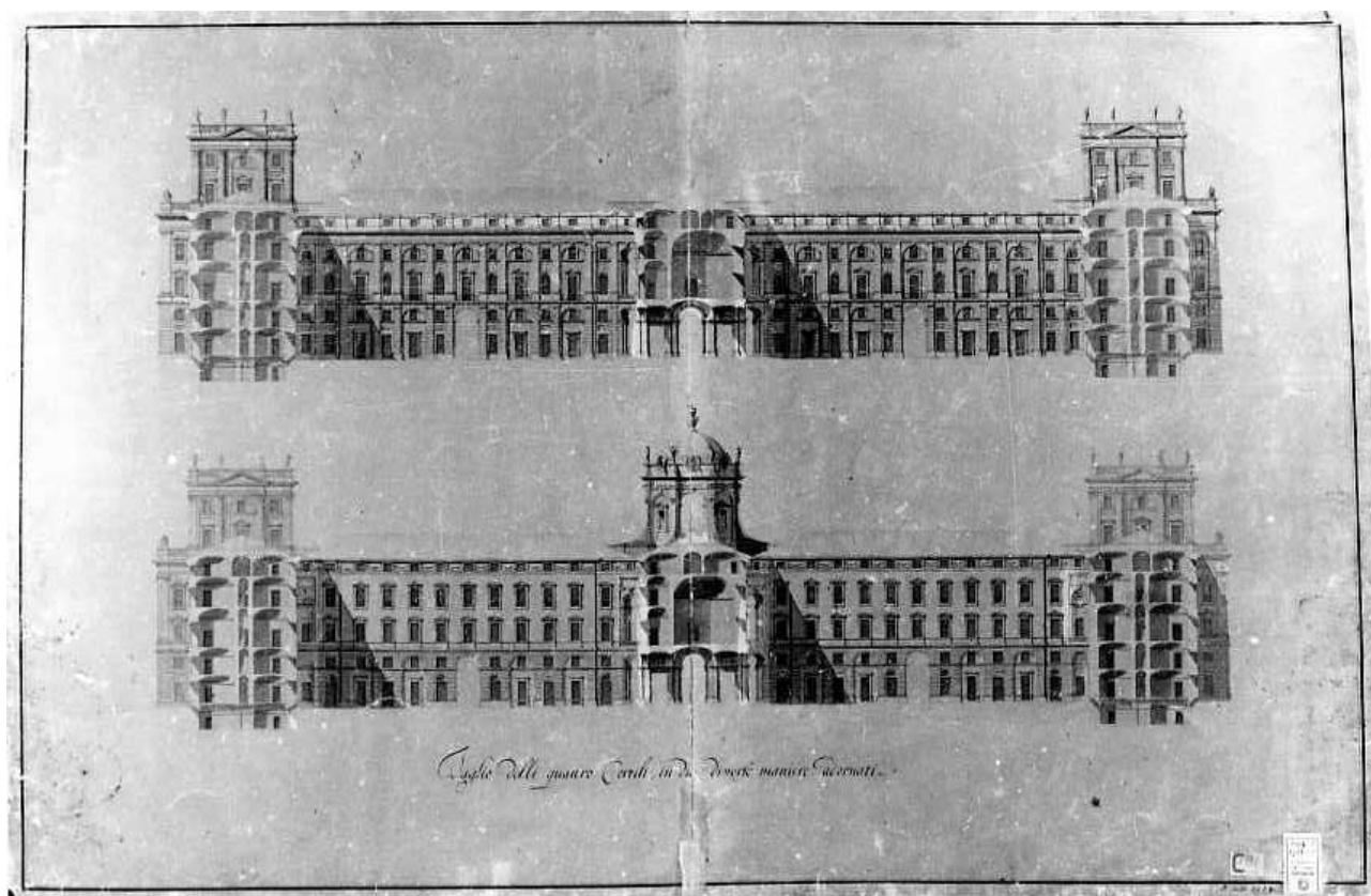
Sezione mediana e trasversale dei cortili della Reggia di Caserta
