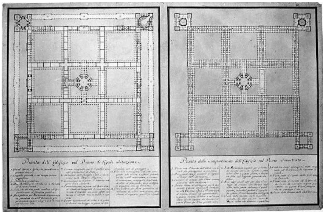
Disegno della pianta dell'edificio nel piano di regale abitazione
