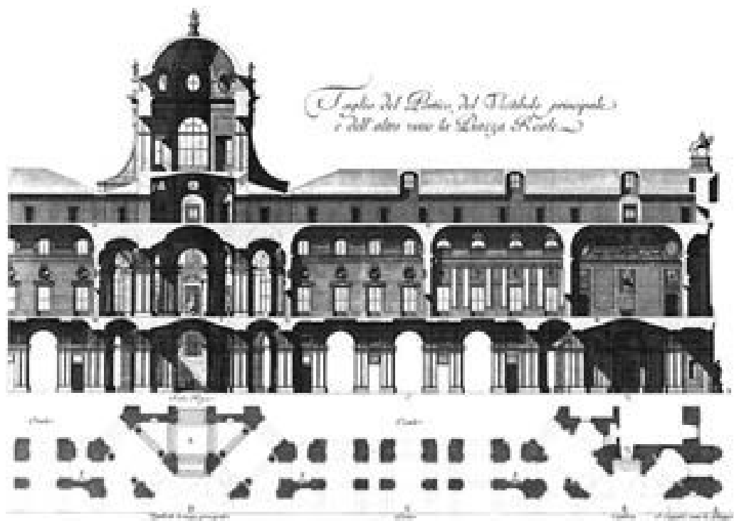
Taglio del portico, del vestibolo principale e dell'altro verso la piazza reale
