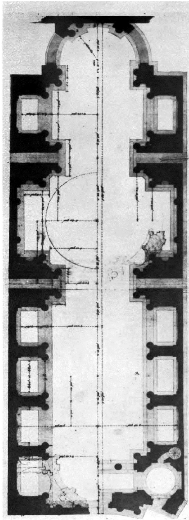
Pianta della chiesa dell'Annunziata Napoli
