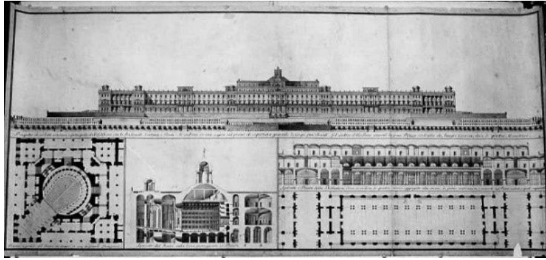
Reggia di Caserta, Prospetto di un lato dell'edificio; pianta del teatro; spaccato del teatro; spaccato e pianta della Biblioteca
