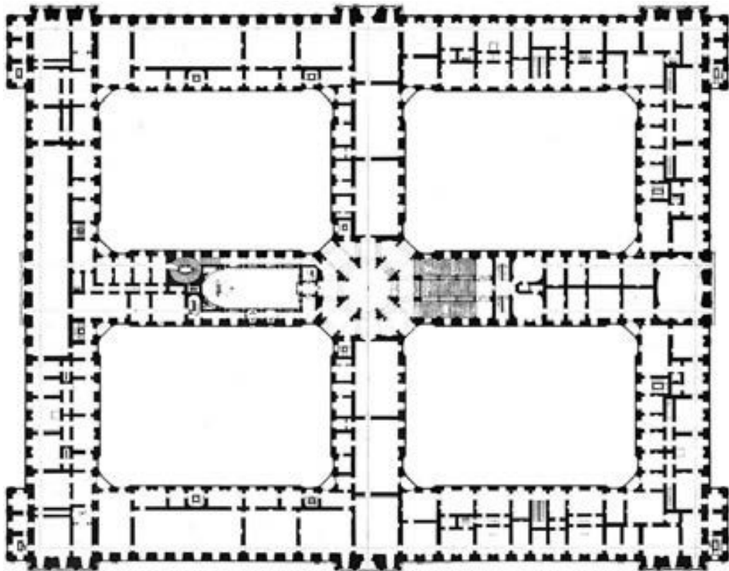
Dichiarazione dei disegni, elaborati del prospetto del Real Palazzo di Caserta: Pianta del piano nobile
