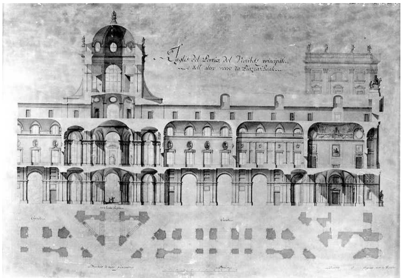
Sezione longitudinale mediana della Reggia
