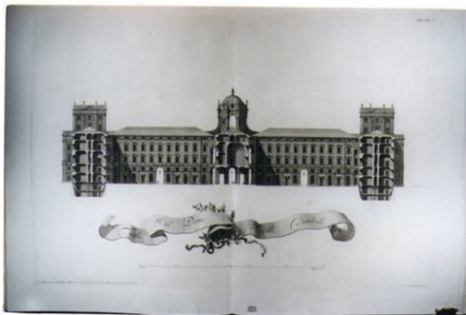
Pianta dell'alzato e portico dei cortili della Reggia di Caserta
