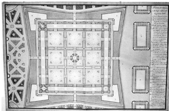
Disegno della pianta dell'edificio e dei corpi adiacenti a piano terra (dai progetti per la Reggia di Caserta)
